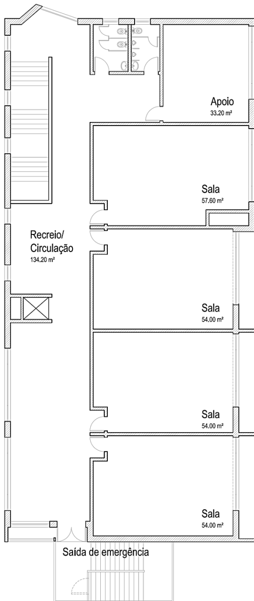
Piso 1
