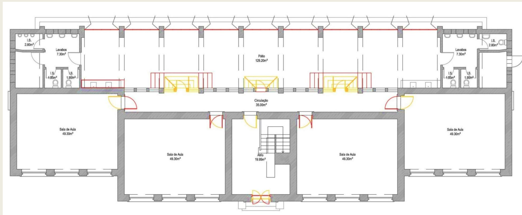
Piso 0
