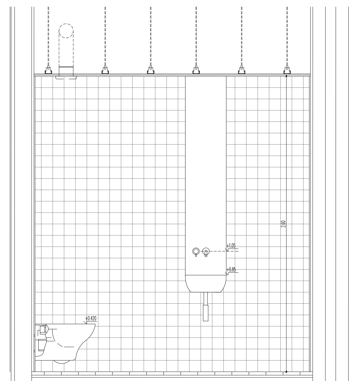
corte 01 esc. 1/20 @A1
