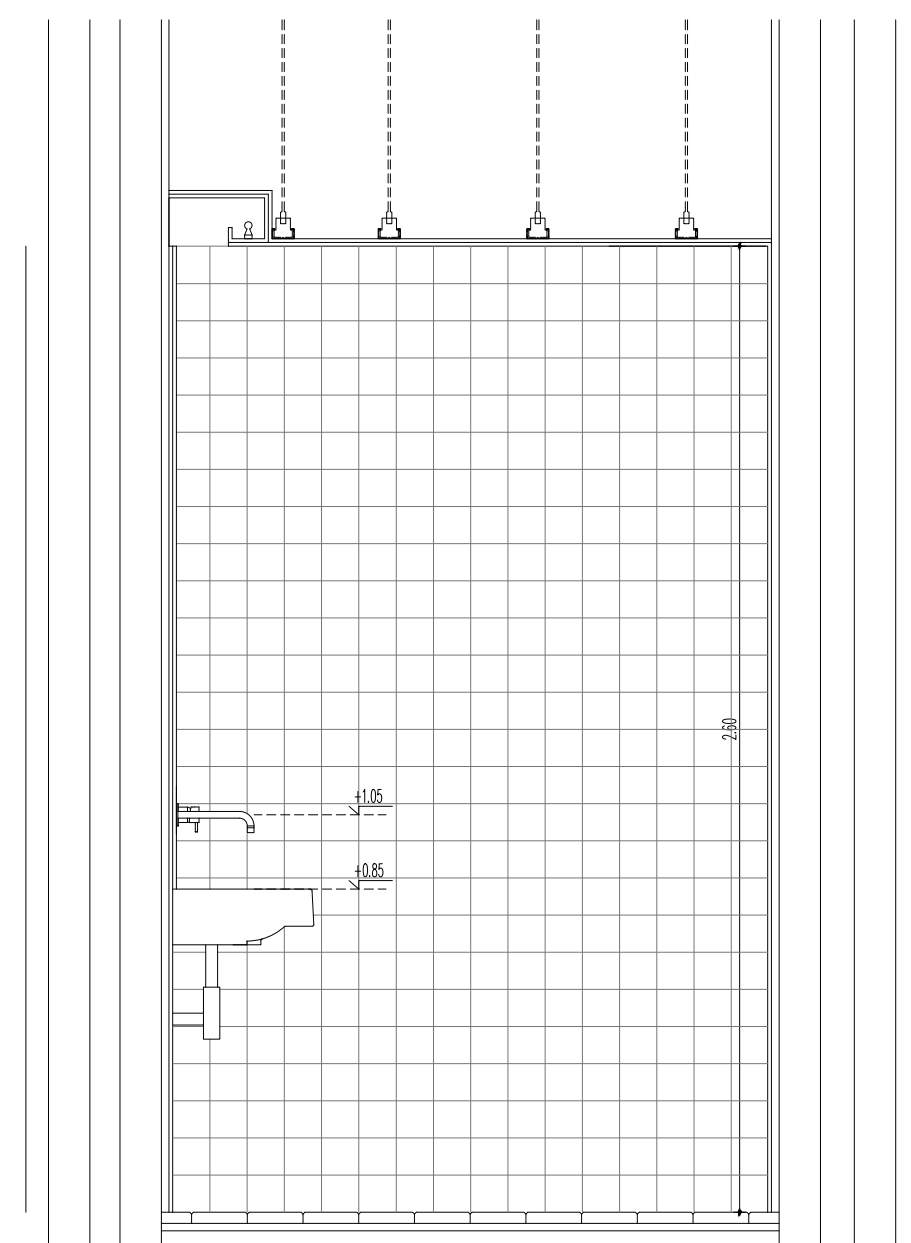
corte 03 esc. 1/20 @A1
